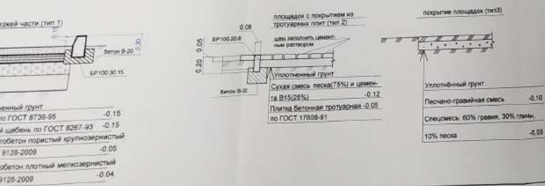
Конструктивные разрезы, М 1:50
