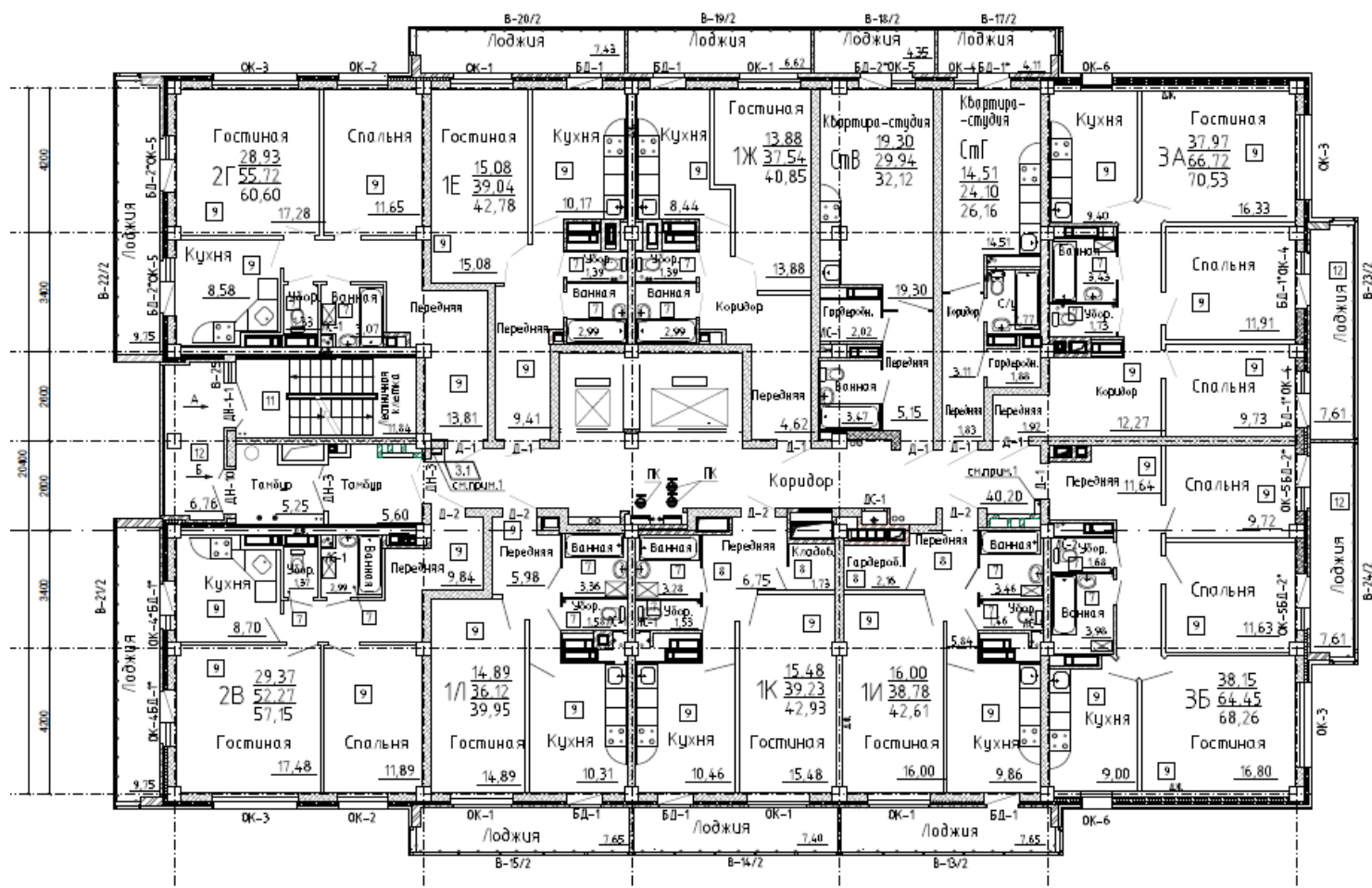
План типового этажа
