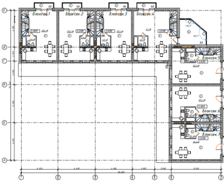
План этажа на отм. 3,000
