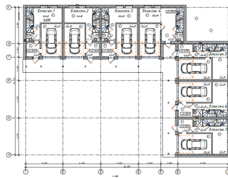
План этажа на отм. 0,000
