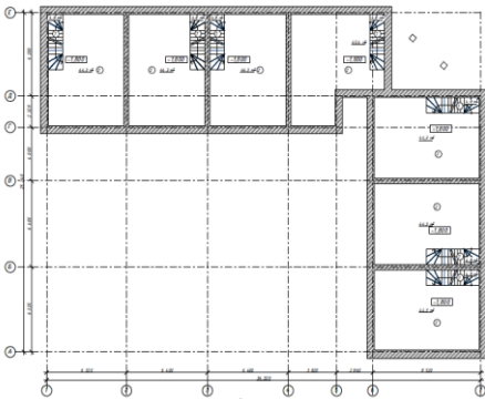
План этажа на отм. -1,800
