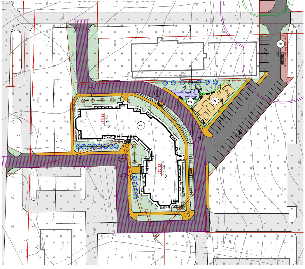
Схема планировочной организации земельного участка М 1:400
