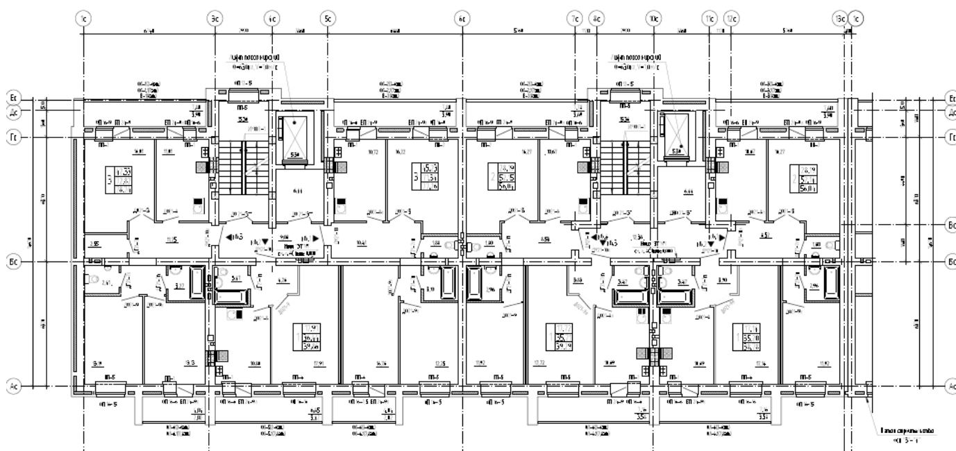
Отделочный план типового этажа
