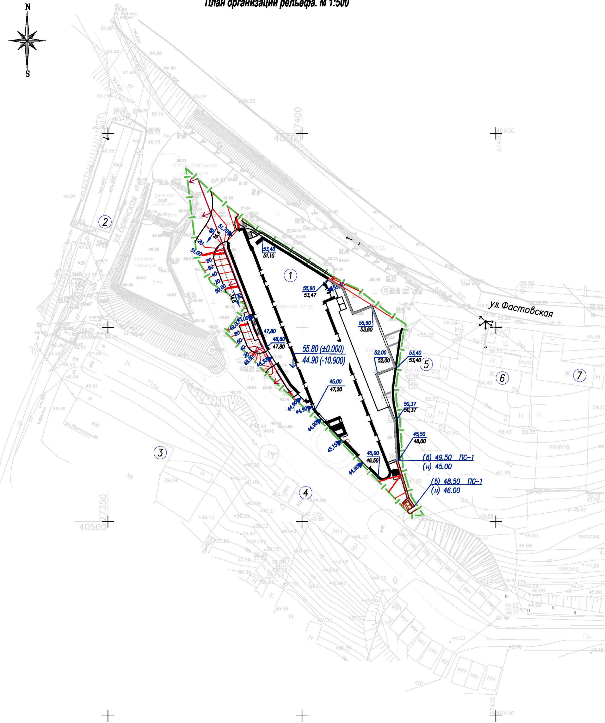
План организации рельефа. М 1:500
