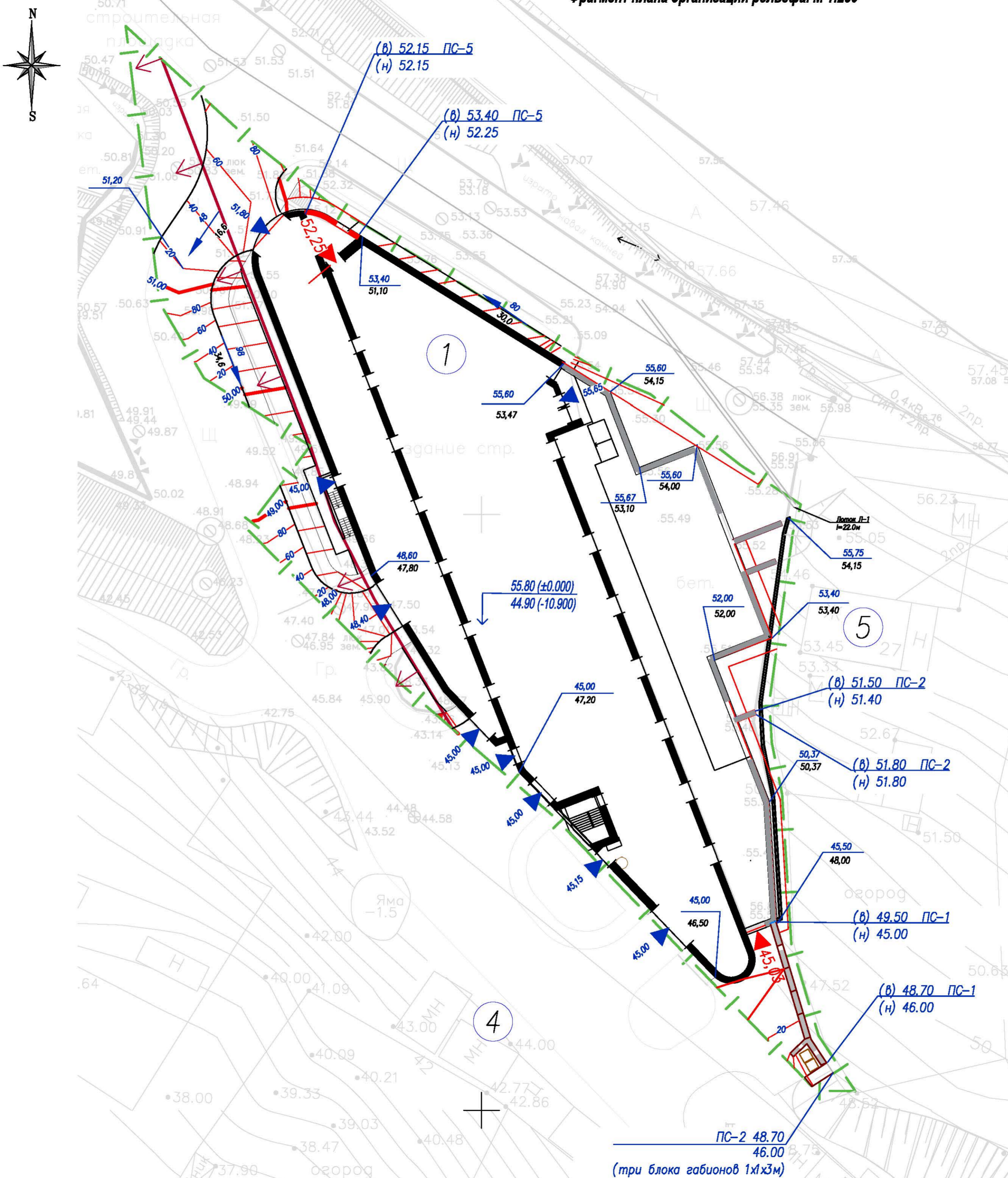
Фрагмент плана организации рельефа. М 1:250
