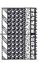
Тип 4 Конструкция дорожных одежд проездов
