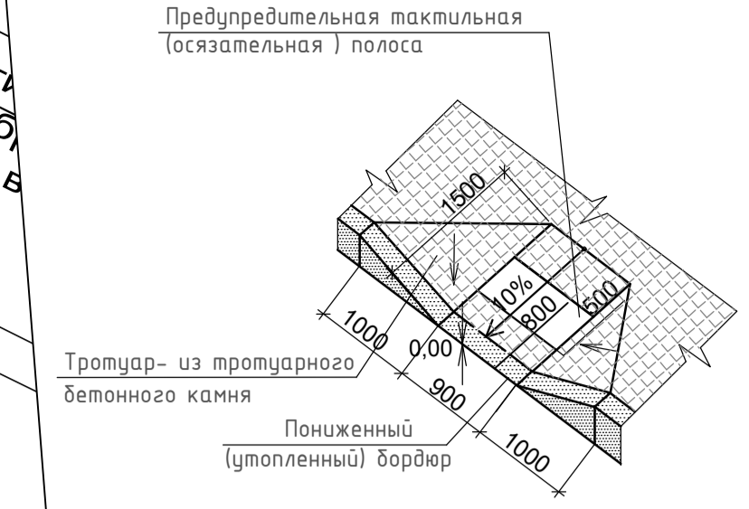
ДЕТАЛЬ УСТРОЙСТВА Пониженного бордюра Б2
