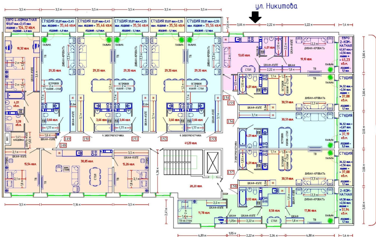
ПЛАН 2-ГО ЭТАЖА (1 ОЧЕРЕДЬ).
