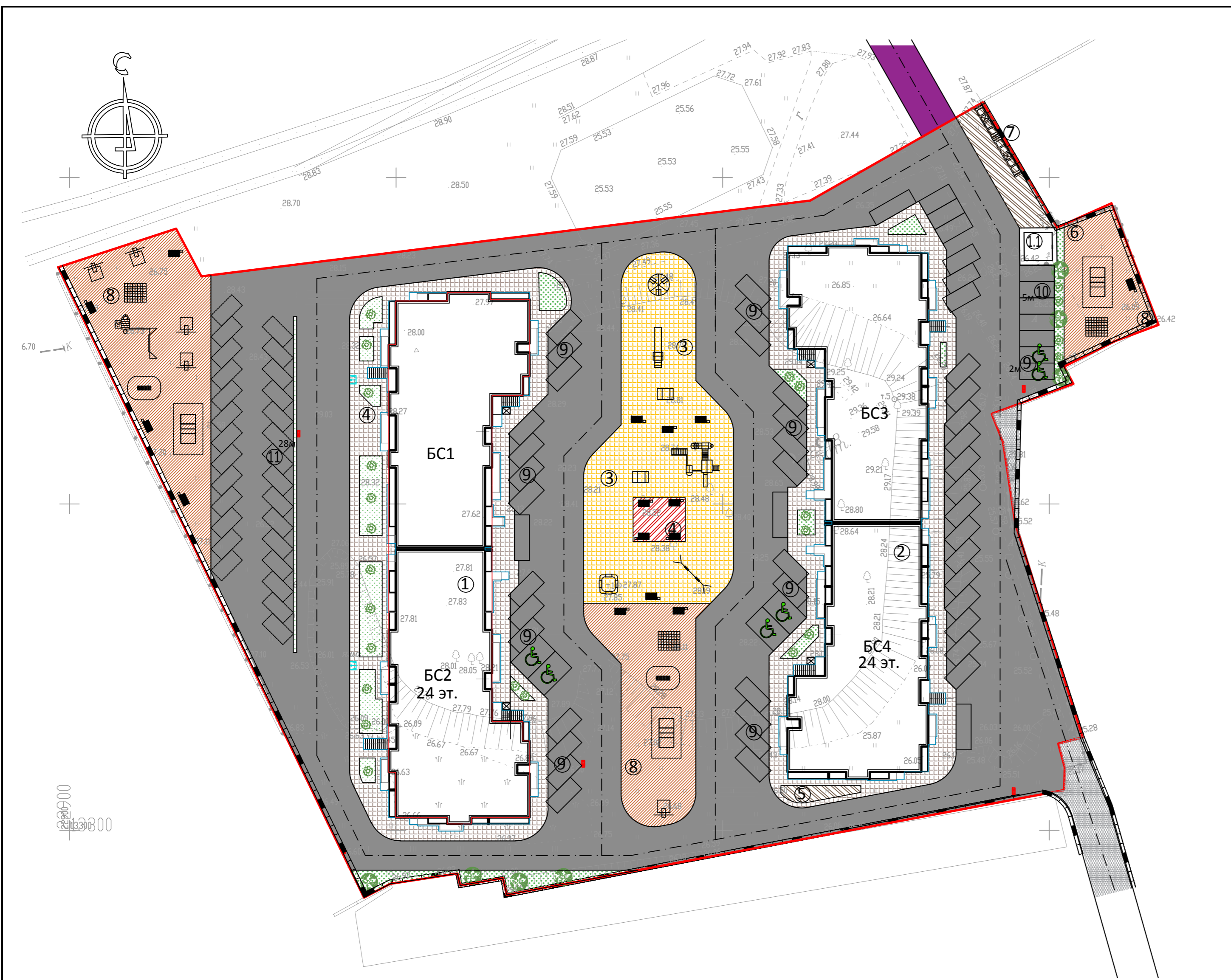
ВЕДОМОСТЬ ПОКРЫТИЙ
