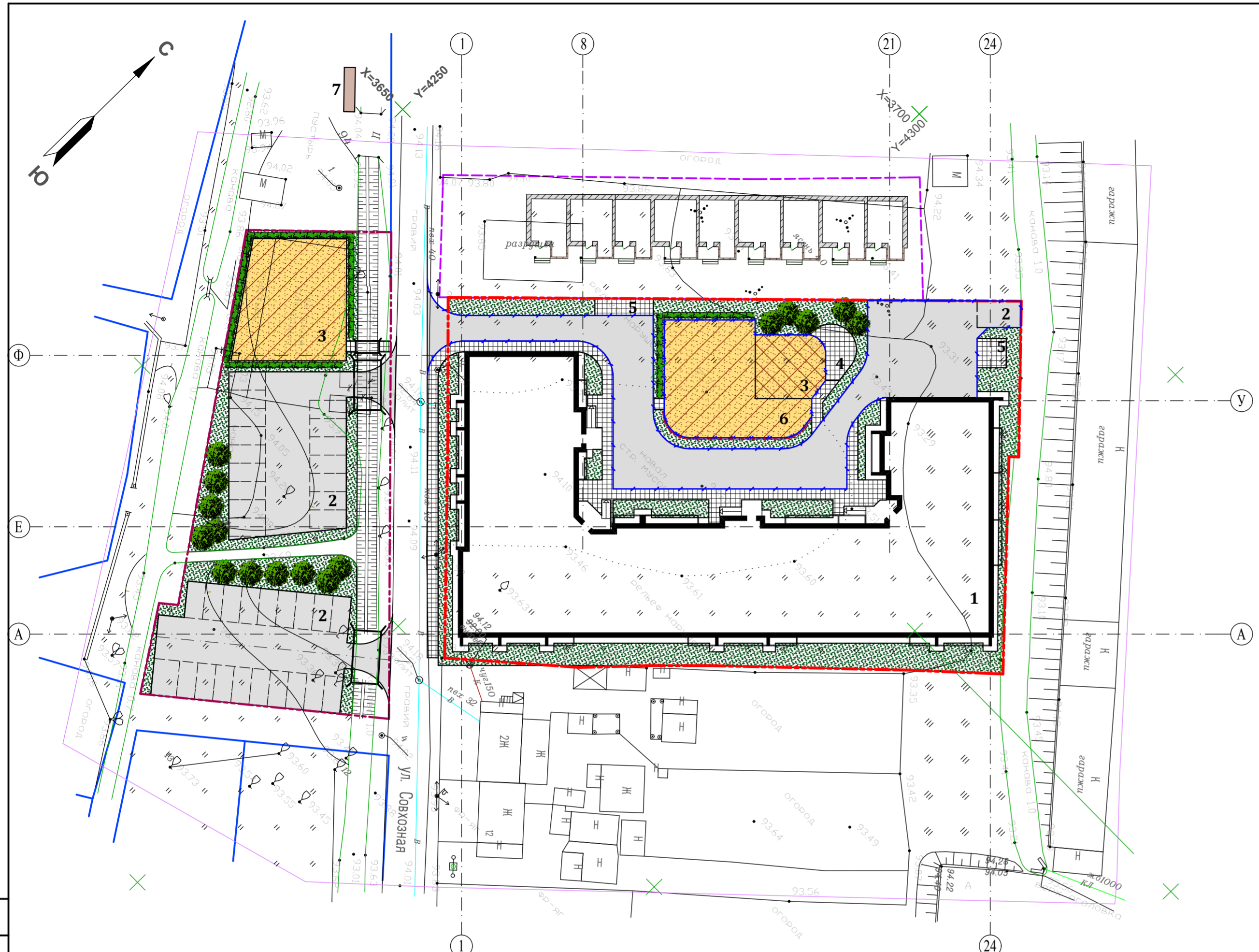
Расстановка малых форм архитектуры на детской, физкультурной площадке и площадке для отдыха
