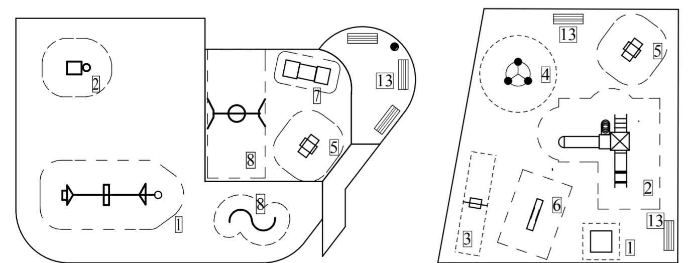
Расстановка малых форм архитектуры на детской, физкультурной площадке и площадке для отдыха
