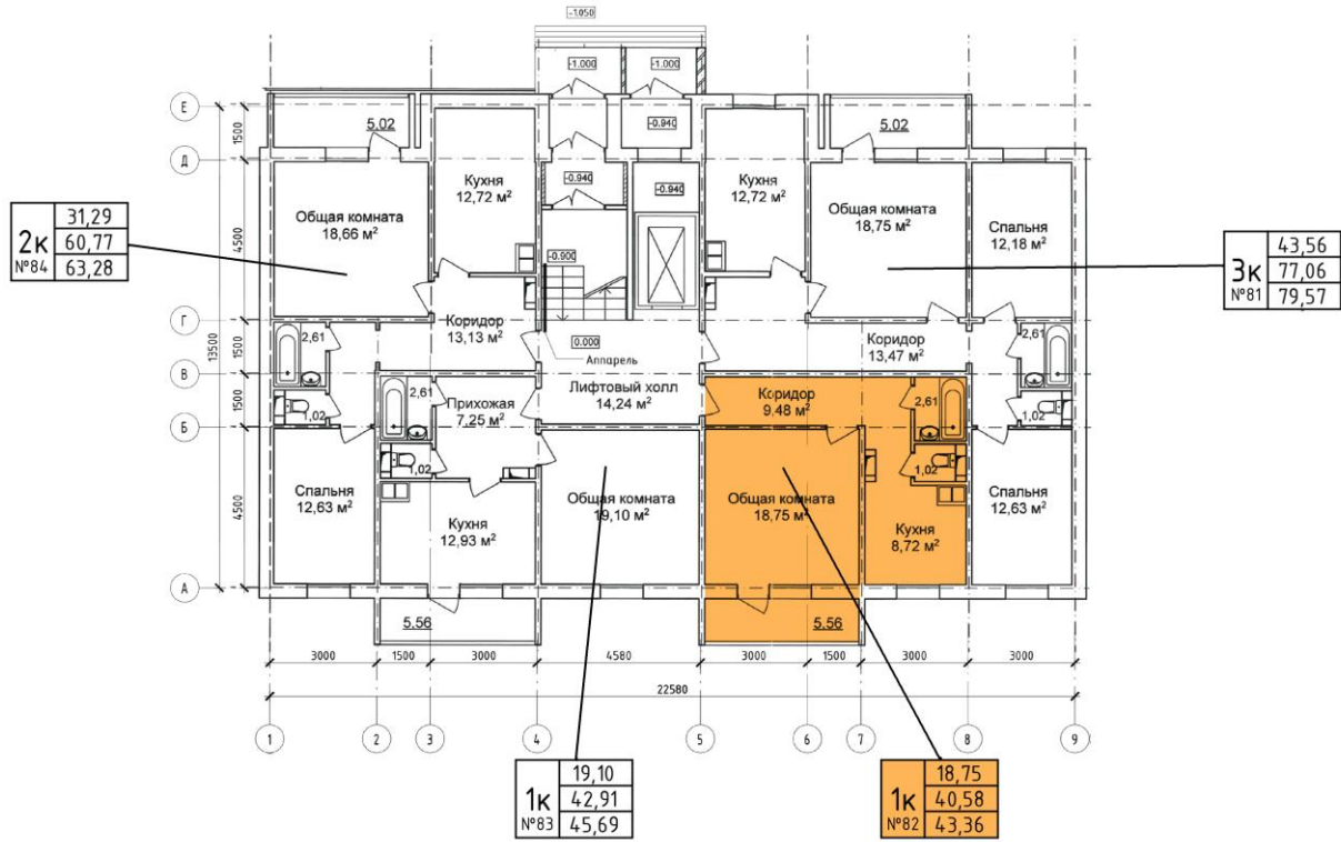
Экспликация к поэтажному плану здания (строения)
