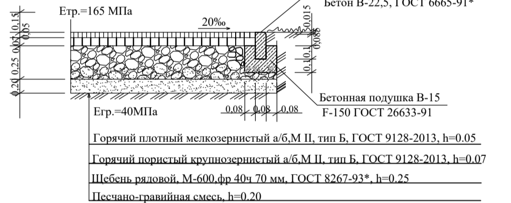
Деталь детских и спортивных площадок ТИП -4
