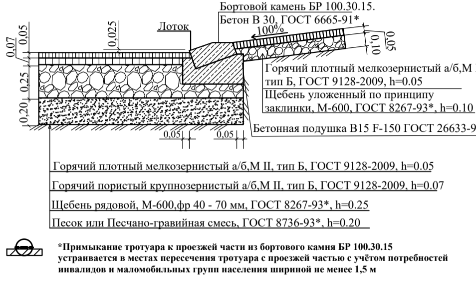
Примыкание тротуара из а/б к проезжей части (с учётом потребностей инвалидов и маломобильных групп населения)*
