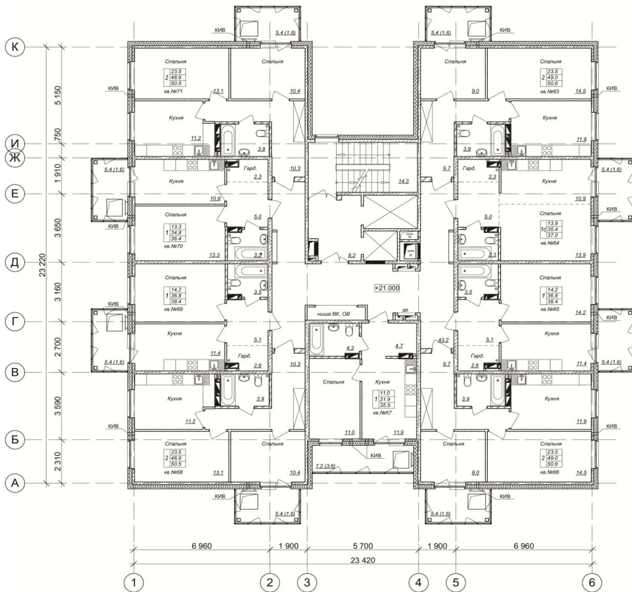
Экспликация к поэтажному плану здания (строения)
