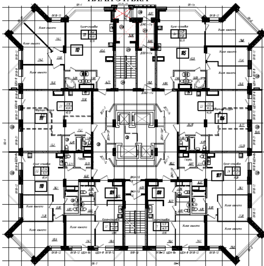
ПЛАН ЭТАЖА
