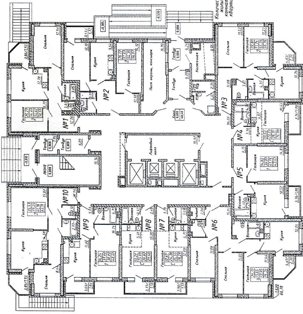
План 1-го этажа от м. 0,000
