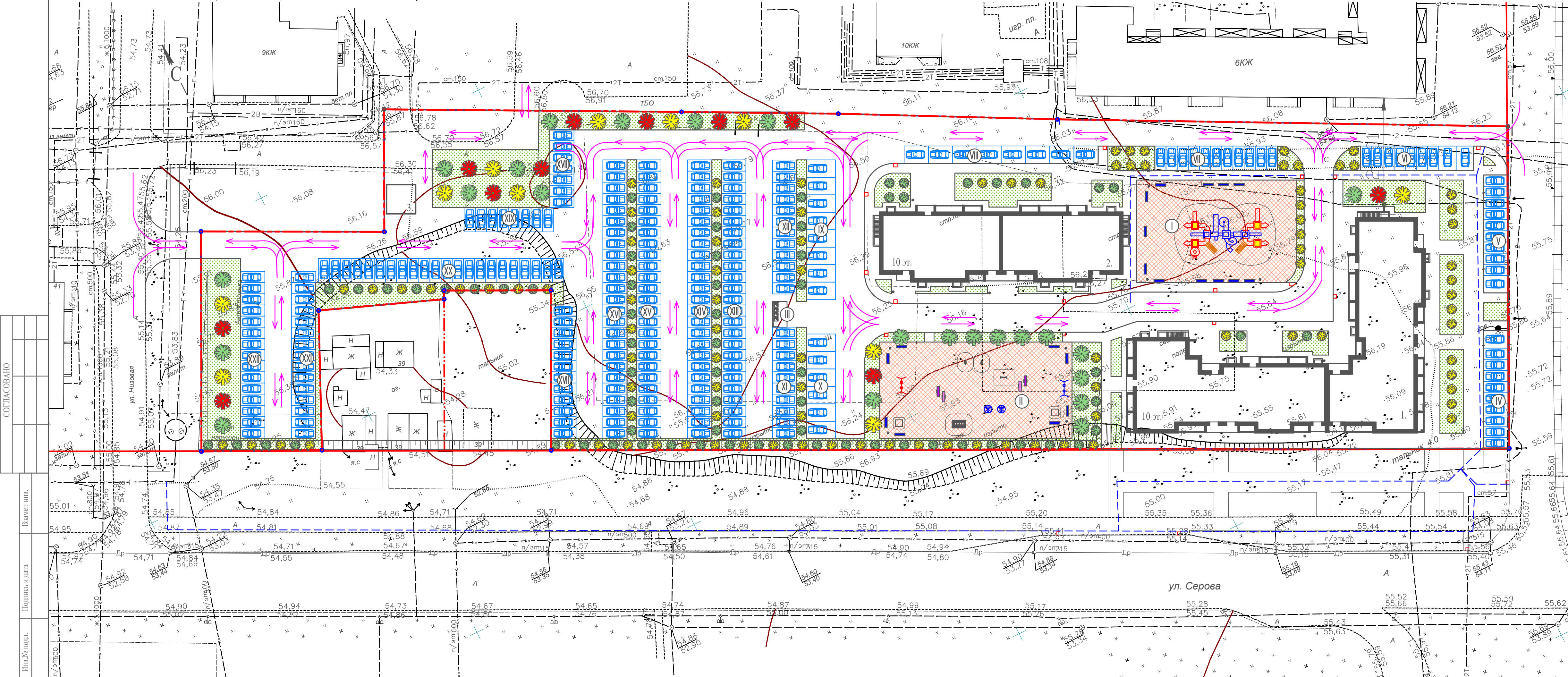
Схема планировочной организации земельного участка М 1:500.
